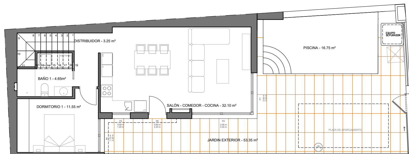
PLANTA BAJA
